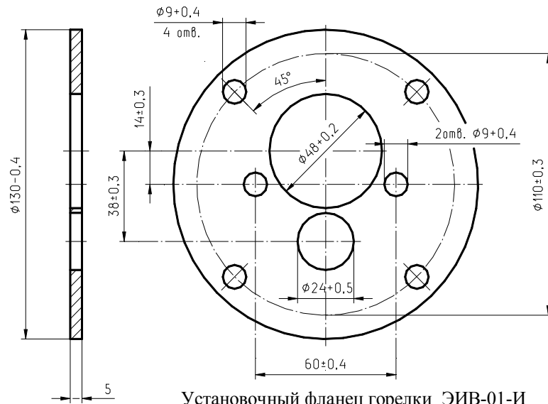
Установочный фланец горелки ЭИВ-01-И
