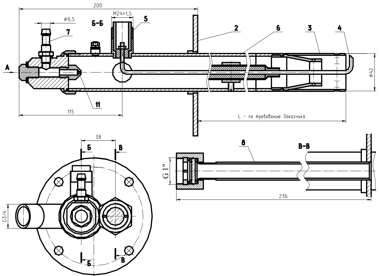
Горелка запальная ЭИВ-01-ДФ
