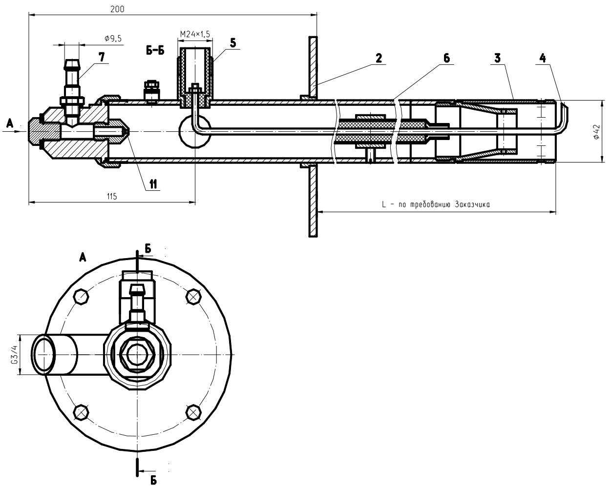
Горелка запальная ЭИВ-01-Д
